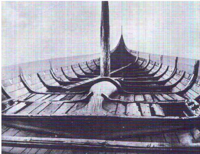
Figura 1.4. Navío vikingo desenterrado en Oseberg (Noruega)
