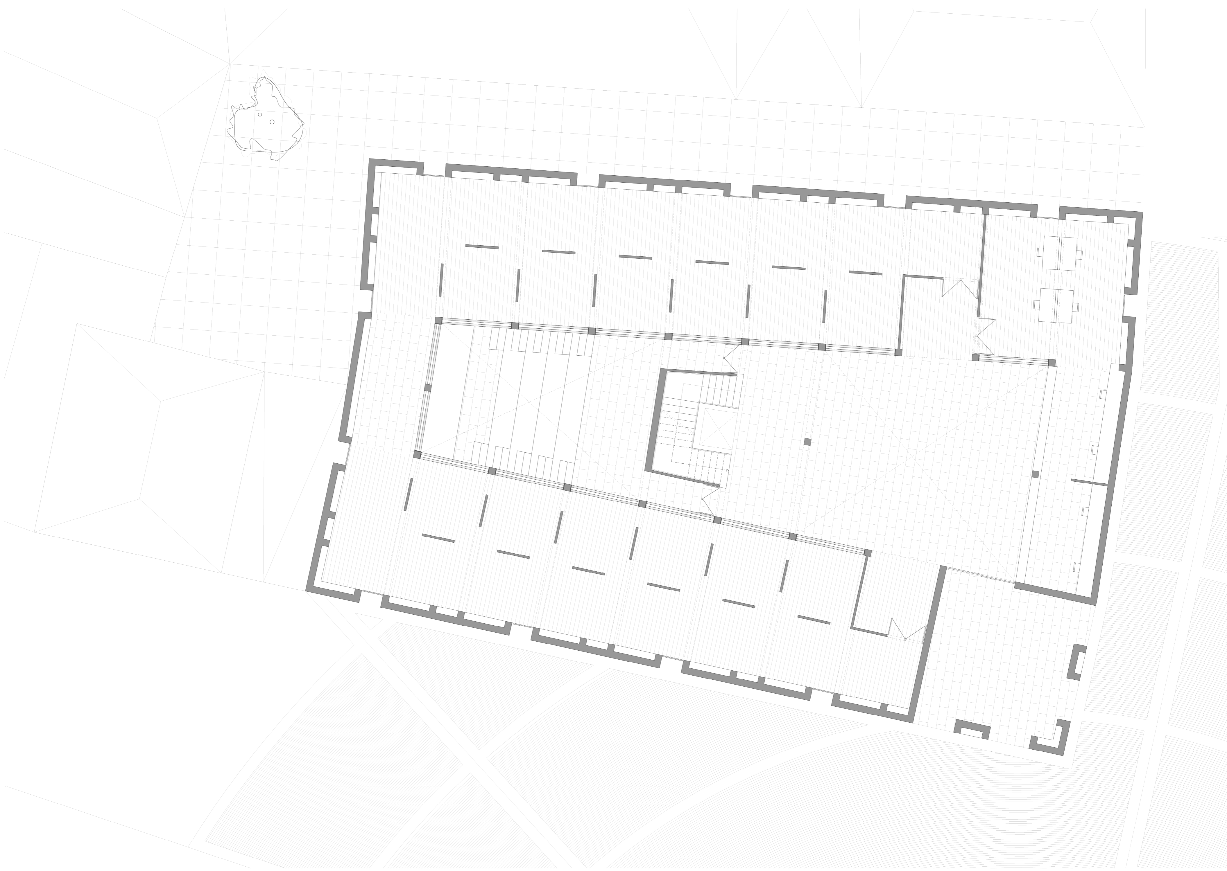
Planta baja E 1:100 m
