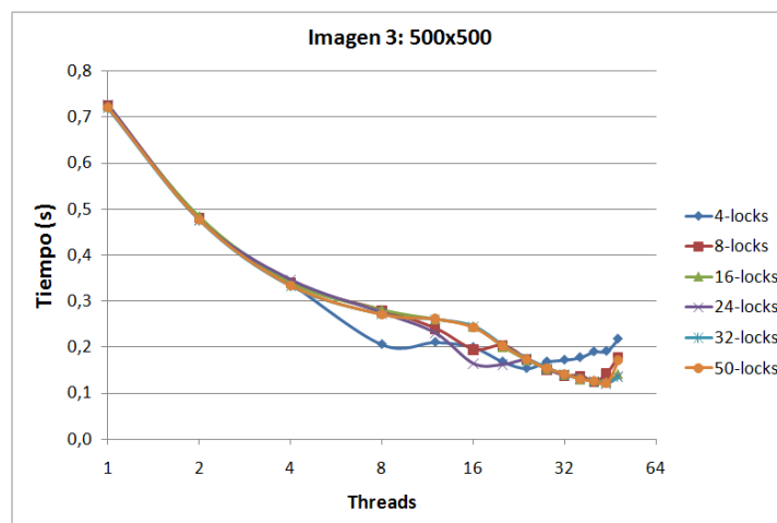
Figura 7.10: Gráfica de los tiempos de ejecución de la imagen 7.1c con un tamaño de 500x500
