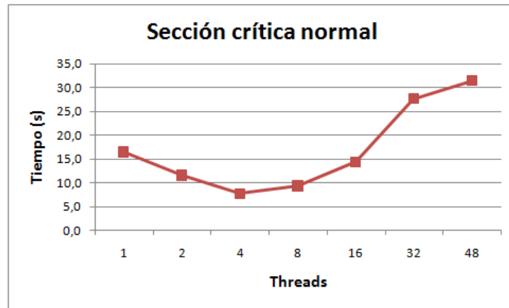
Figura 6.7: Gráfica de los tiempos de ejecución de la primera implementación paralela
