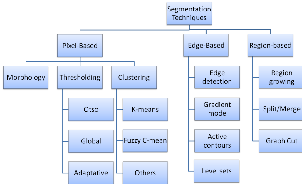
Figura 3.1: Clasificación de las técnicas de segmentación
