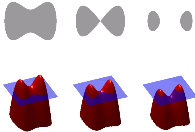
Figura 3.13: Ilustración del método level set
