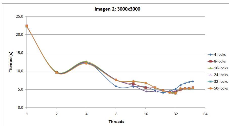
Figura 7.8: Gráfica de los tiempos de ejecución de la imagen 7.1b con un tamaño de 3000x3000
