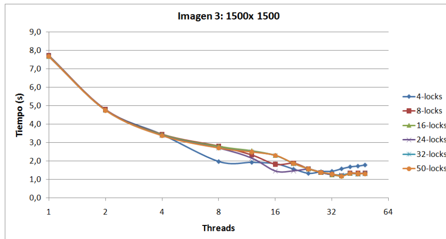
Figura 7.11: Gráfica de los tiempos de ejecución de la imagen 7.1c con un tamaño de 1500x1500
