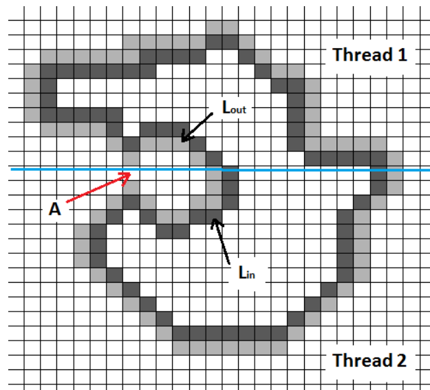
Figura 6.1: Ejemplo de condición de carrera al querer añadir un punto vecino en común a puntos tratados por distintos threads
