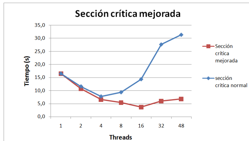
Figura 6.8: Gráfica de los tiempos de ejecución de la primera y segunda implementación
