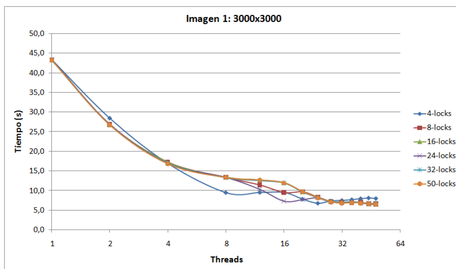
Figura 7.4: Gráfica de los tiempos de ejecución de la imagen 7.1a con un tamaño de 3000x3000
