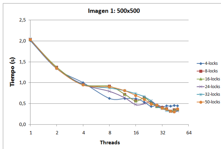
Figura 7.2: Gráfica de los tiempos de ejecución de la imagen 7.1a con un tamaño de 500x500
