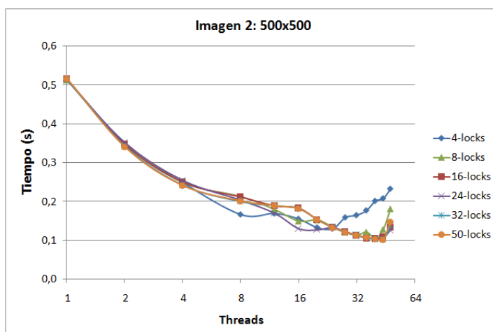
Figura 7.6: Gráfica de los tiempos de ejecución de la imagen 7.1b con un tamaño de 500x500
