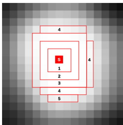
Figura 3.14: Ejemplo del funcionamiento de la técnica de region growing
