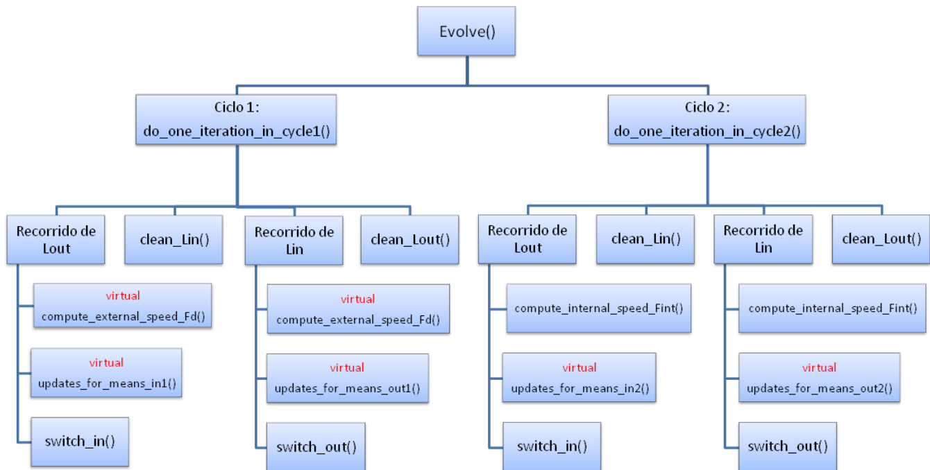
Figura 5.1: Esquema de las funciones utilizadas en el trabajo de Ofeli para realizar el algoritmo level set aproximado
