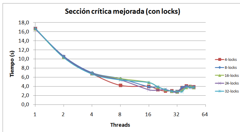
Figura 6.10: Gráfico de los resultados obtenidos en esta tercera implementación
