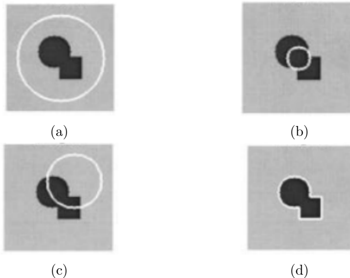
Figura 4.3: Posibles inicializaciones del contorno con el método de Chan-Vese
