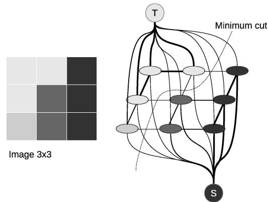
Figura 3.19: Funcionamiento de la técnica de graph cut en una imagen 3x3
