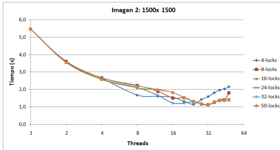
Figura 7.7: Gráfica de los tiempos de ejecución de la imagen 7.1b con un tamaño de 1500x1500
