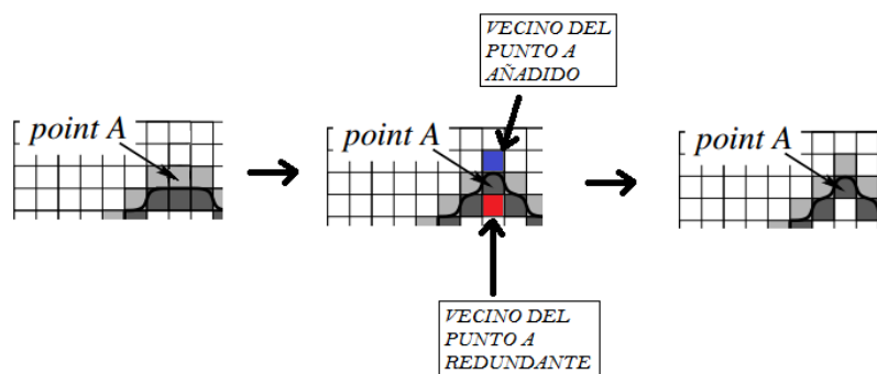
Figura 4.2: Ejemplo de expansión del contorno un píxel hacia fuera. Operaciones que se realizan continuamente en el paso 2 y 3 del algoritmo
