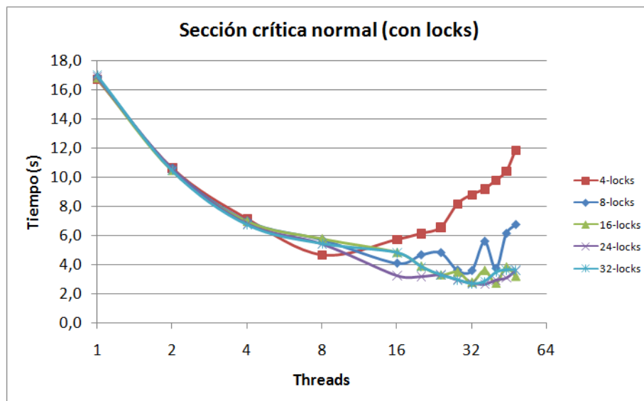
Figura 6.11: Gráfica de los tiempos de ejecución con los locks y la estructura de la «sección crítica normal»
