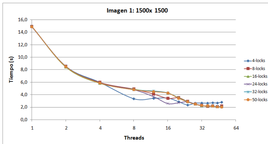
Figura 7.3: Gráfica de los tiempos de ejecución de la imagen 7.1a con un tamaño de 1500x1500
