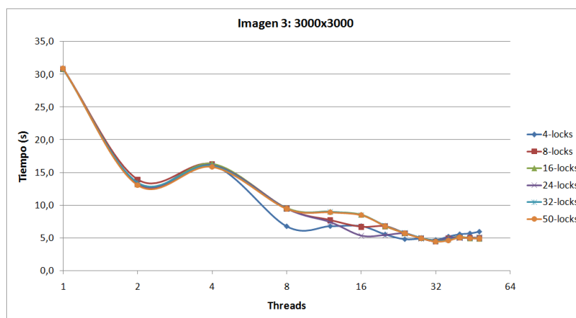
Figura 7.12: Gráfica de los tiempos de ejecución de la imagen 7.1c con un tamaño de 3000x3000
