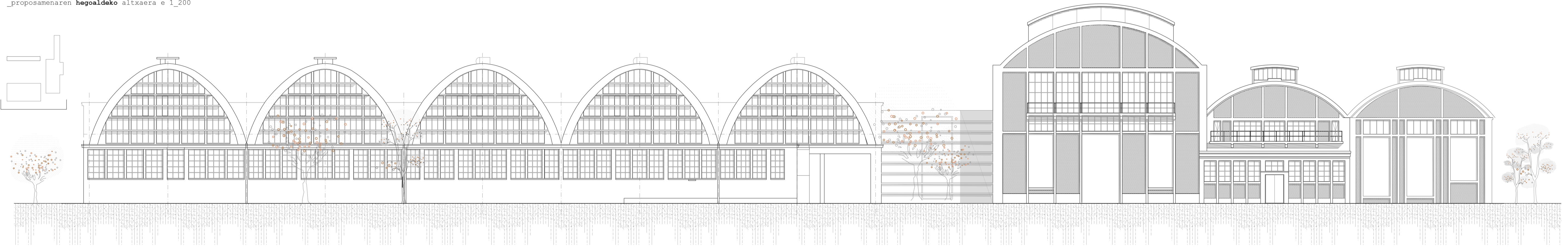
_proposamenaren hegoaldeko altxaera e 1_200
