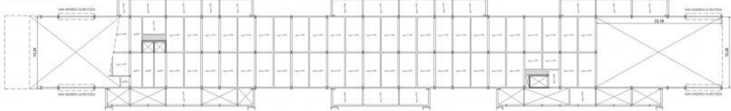
SEZIONE METALICA SEZIONE METALICA TRALICCI QUADRANGOLI E ALTERNATI
