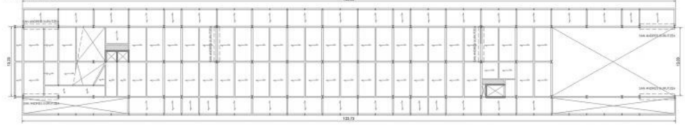
SEZIONE METALICA SEZIONE METALICA TRALICCI QUADRANGOLI E ALTERNATI
