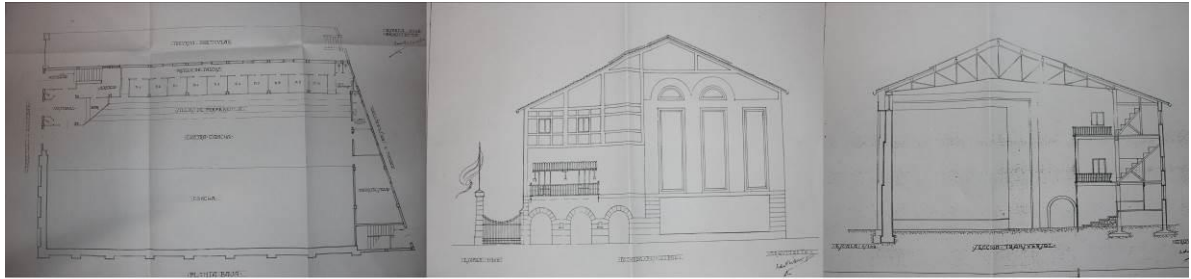
27.Irudia. Gurea Pilotalekuaren planoak (1931). Egilea: Ione Muxika Zuloaga. Iturria: Etxaniz-Iturbe familia.
