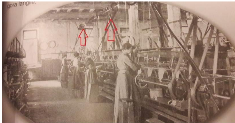
5. Irudia. Hurtado de Mendoza txapel fabrikako makineria. Egilea: Ione Muxika Zuloaga. Iturria: Olalde, 2004: 67
