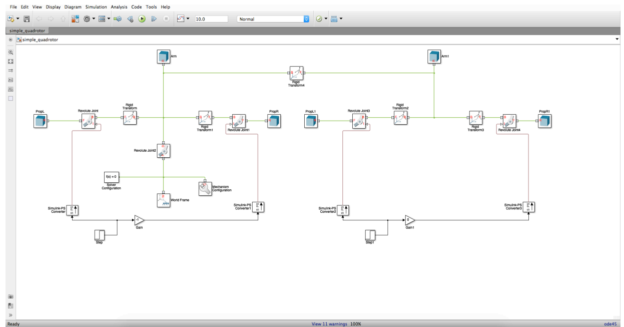
Figura 4.1 Diseño quadrotor simulink.
