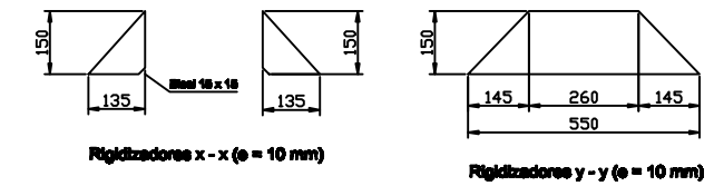
DETALLE 1 RIGIDIZADORES
