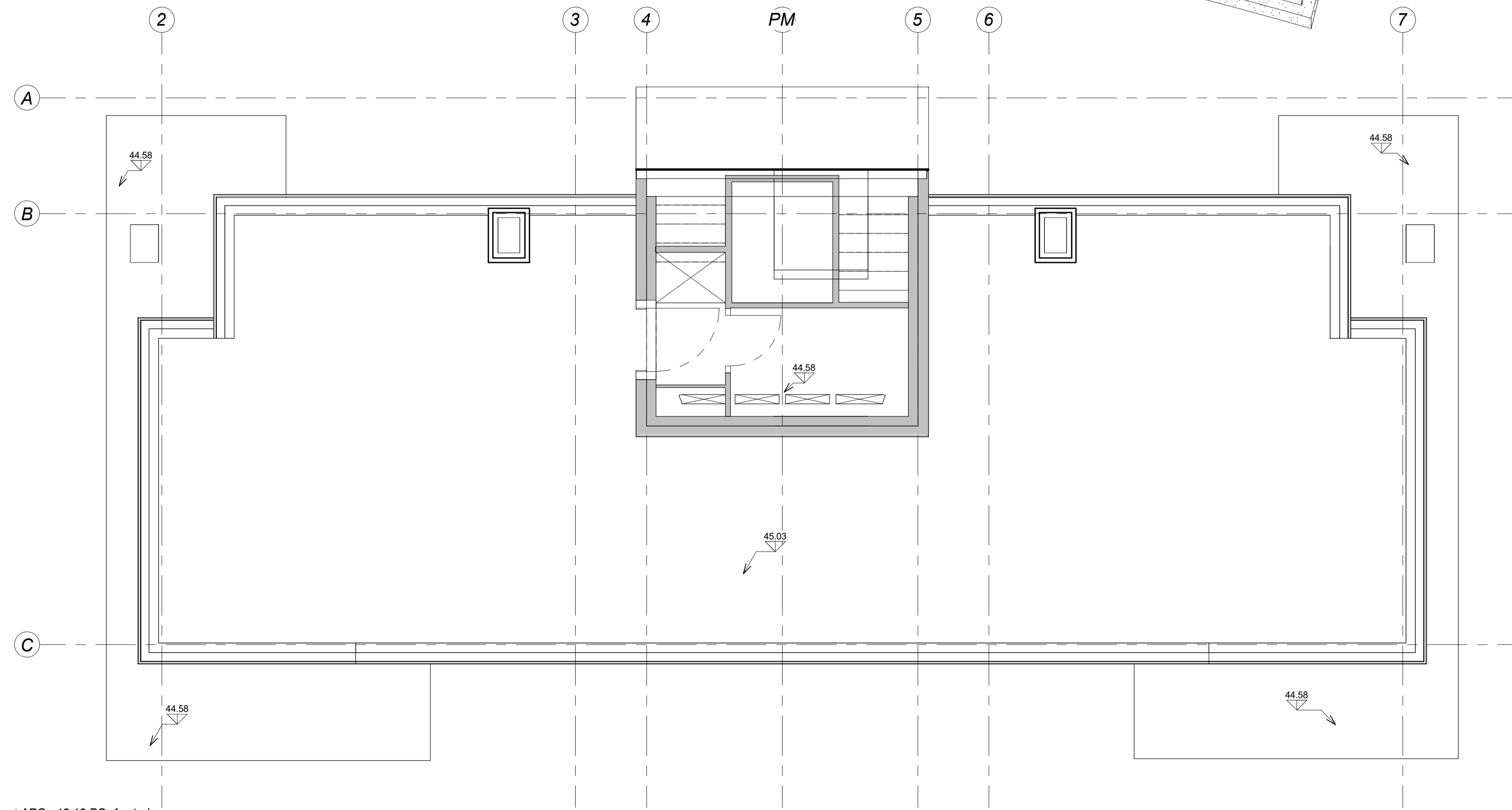
ARQ-06 ARQ +12.18 PC Acotada 1:50
