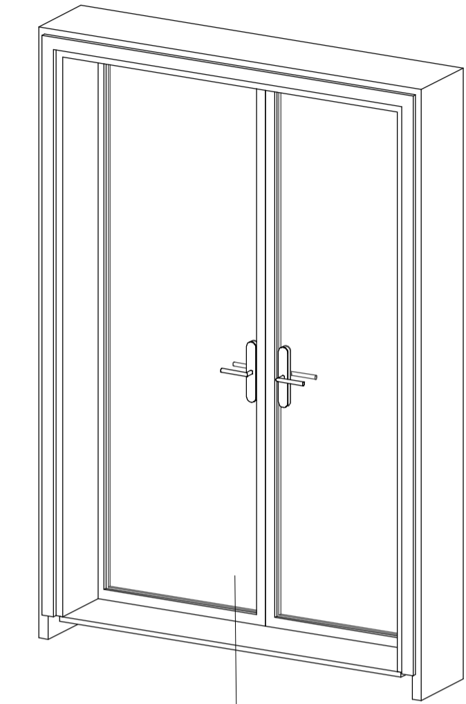
CML_Puerta balconera Alum_225x150 P5 Puerta balconera de aluminio con RPT. Perfiles lacados de blanco.
