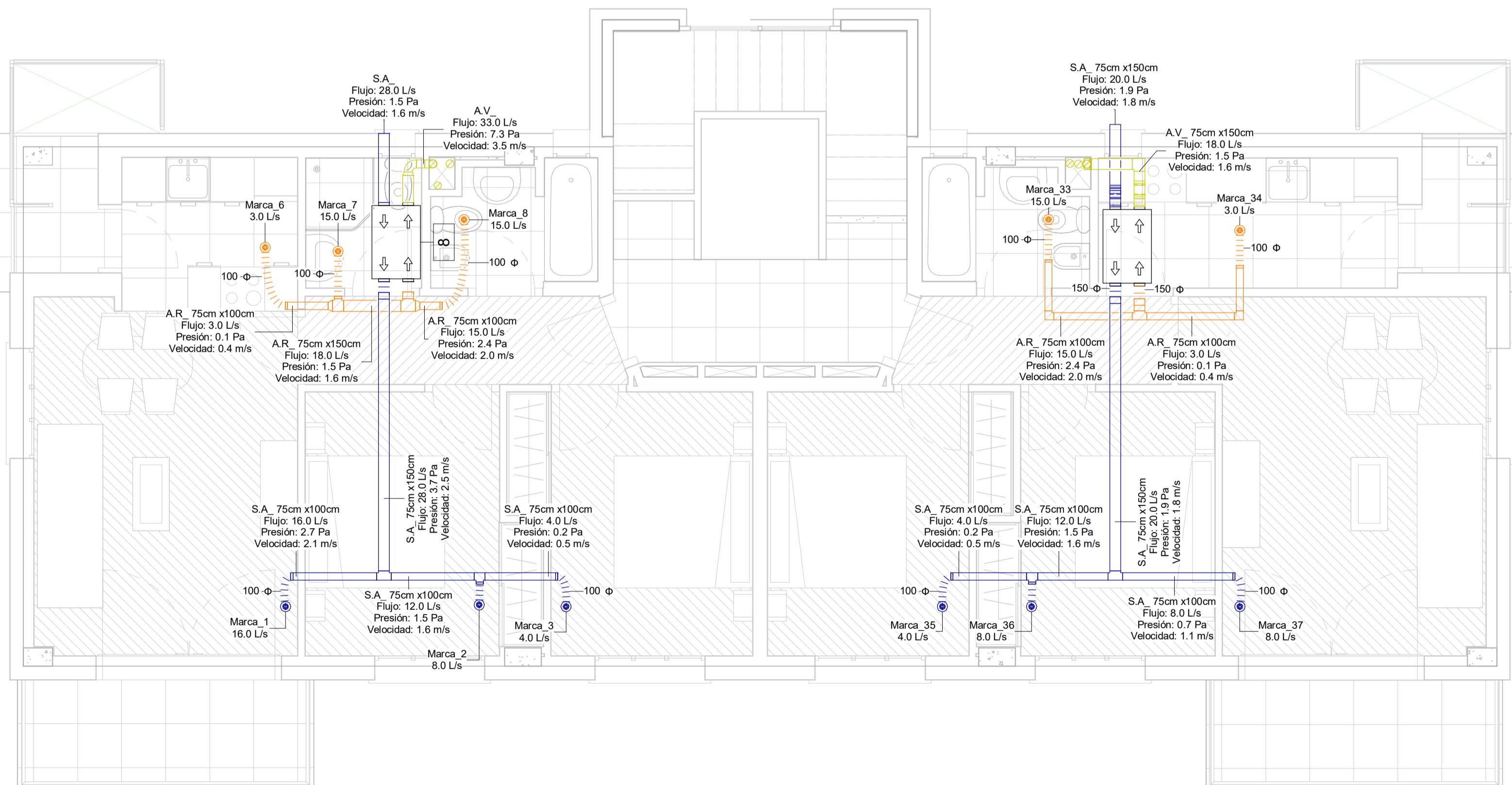
1 Ventilación P3 1 : 50
