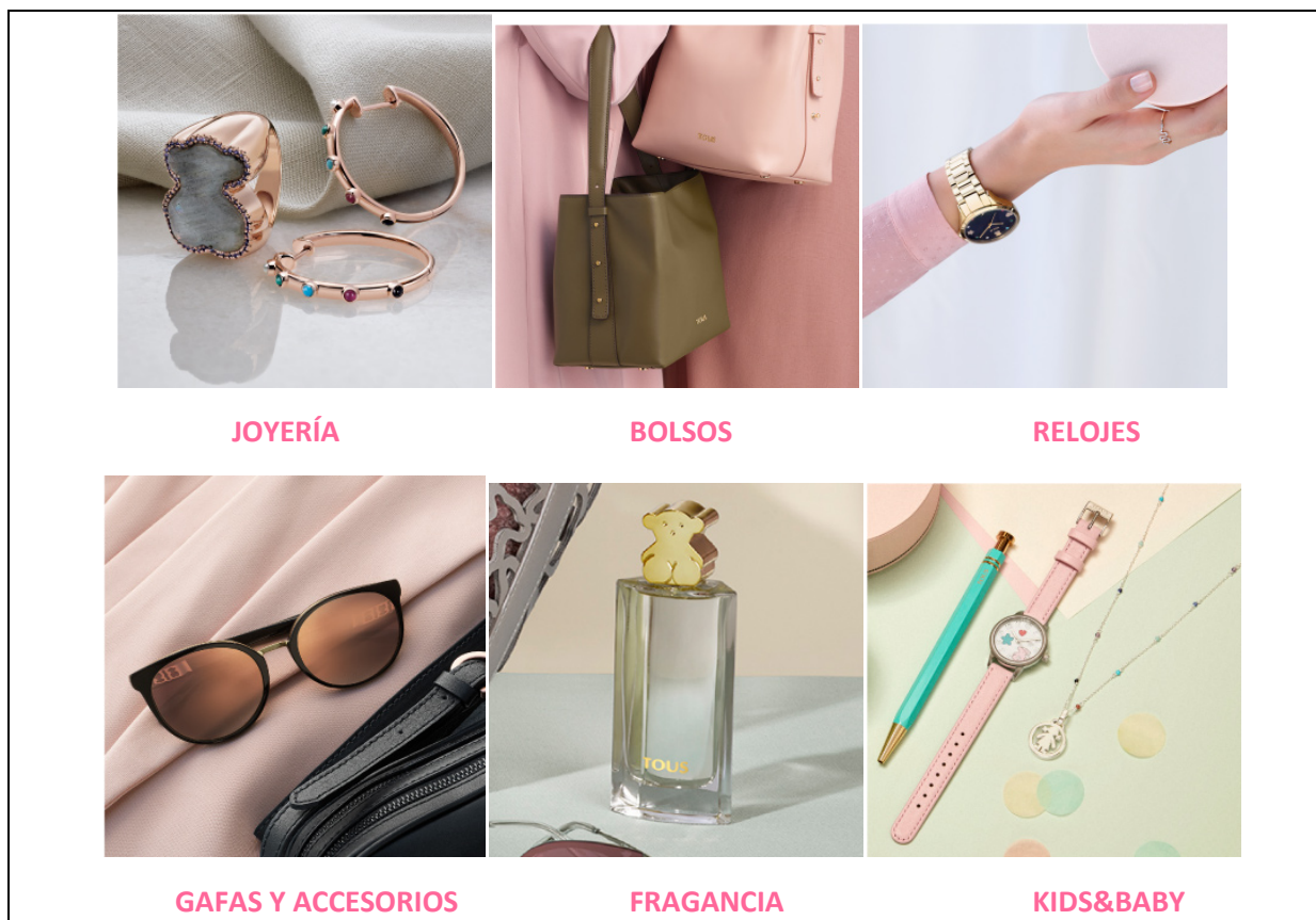
Figura 15: Diversificación
