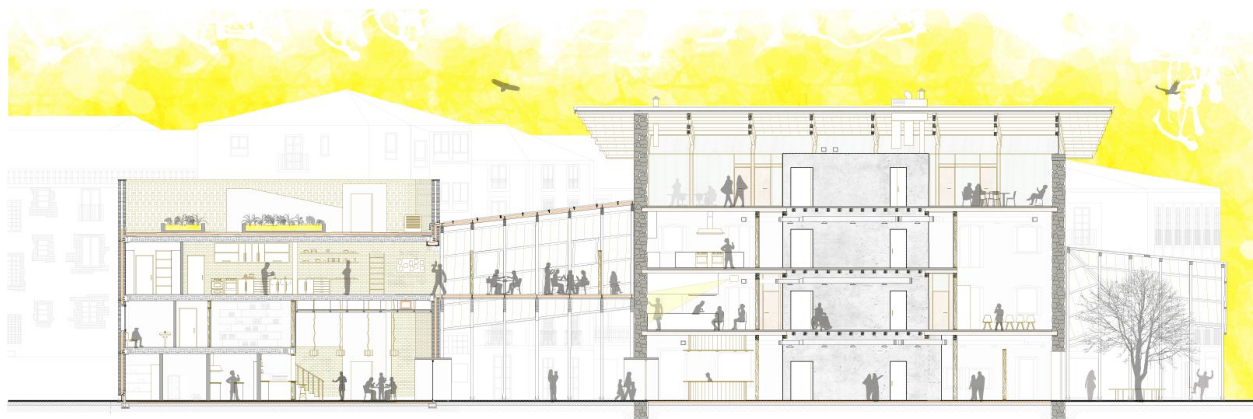
AA' LUZETARAKO EBAKETA
