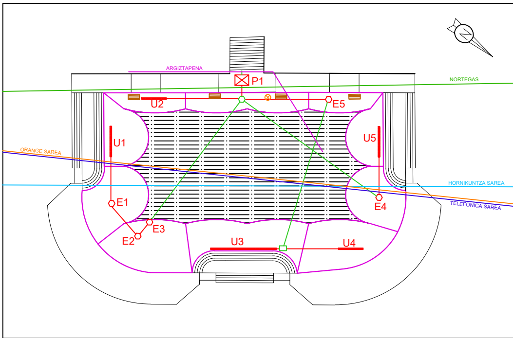
PROPOSATURIKO SOLUZIOA Oinplanta E= 1:500
