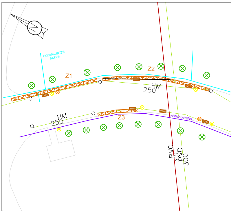
PROPOSATURIKO SOLUZIOA Oinplanta E: 1:500
