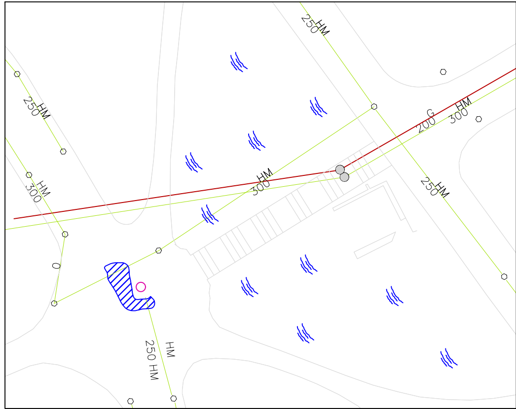
GAUR EGUNGO EGOERA Oinplanta E: 1:500
