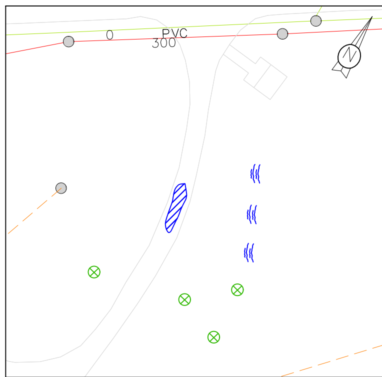
GAUR EGUNGO EGOERA Oinplanta E: 1:500
