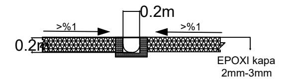
UBIDE DRAINATZAILEA E-E' Zeharkako sekzioa E= E/G
