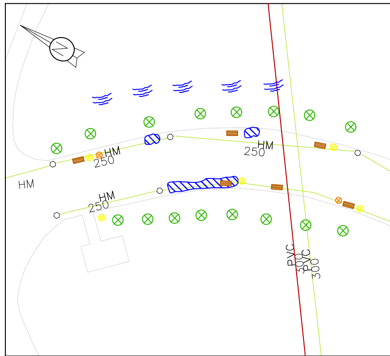
GAUR EGUNGO EGOERA Oinplanta E: 1:500
