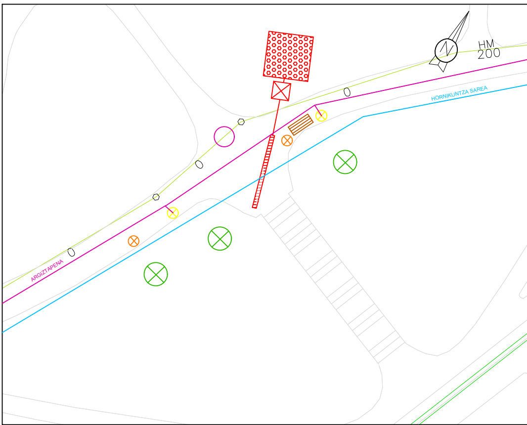
PROPOSATURIKO SOLUZIOA Oinplanta E: 1:500
