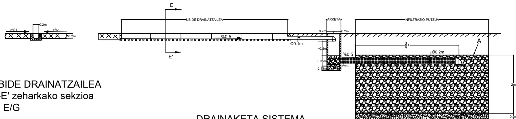
DRAINAKETA SISTEMA Luzetarako profila E: E/G
