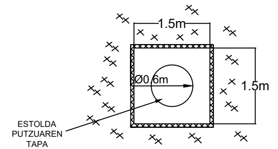
INFILTRAZIO PUTZUA Goitiko bista E= E/G
