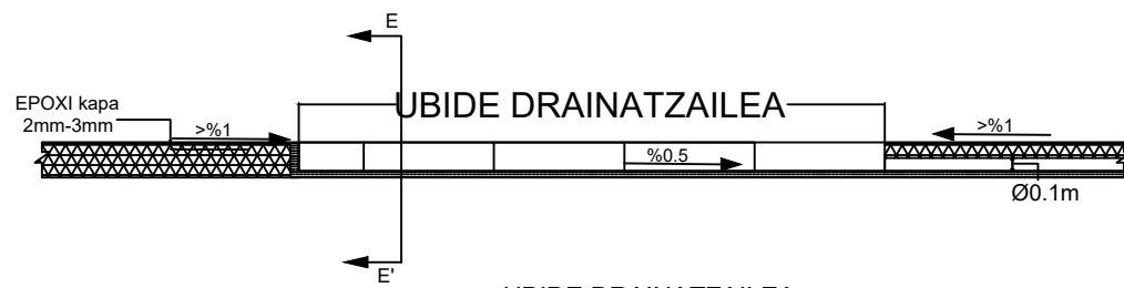
UBIDE DRAINATZAILEA Luzetarako profila E= E/G
