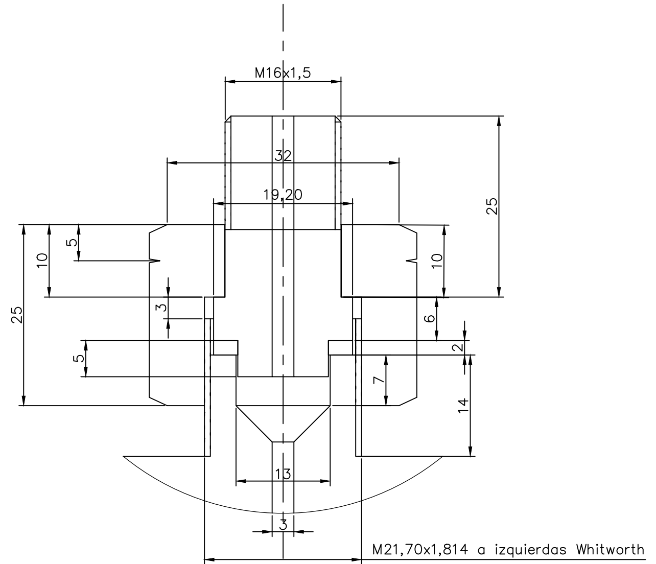
DETALLE ESCALA 2:1 Acoplamiento tipo E para productos inflamables
