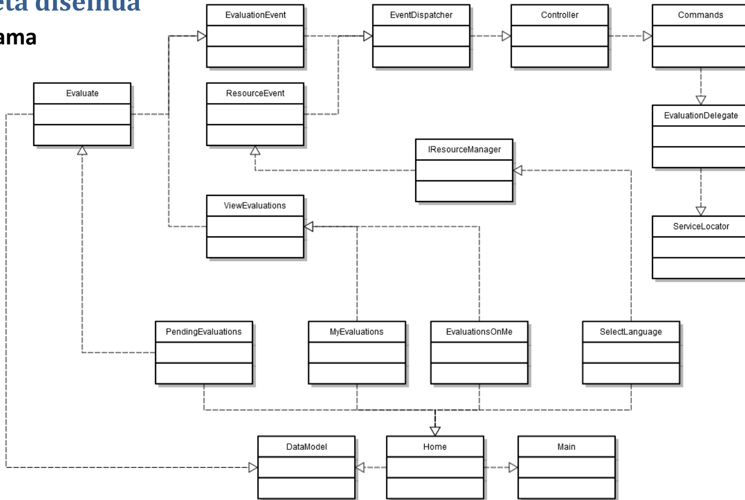
31. irudia: Klase diagrama. "Commands" klasean komando-klase guztiak sartzen dira, exekututzen denaren arabera
