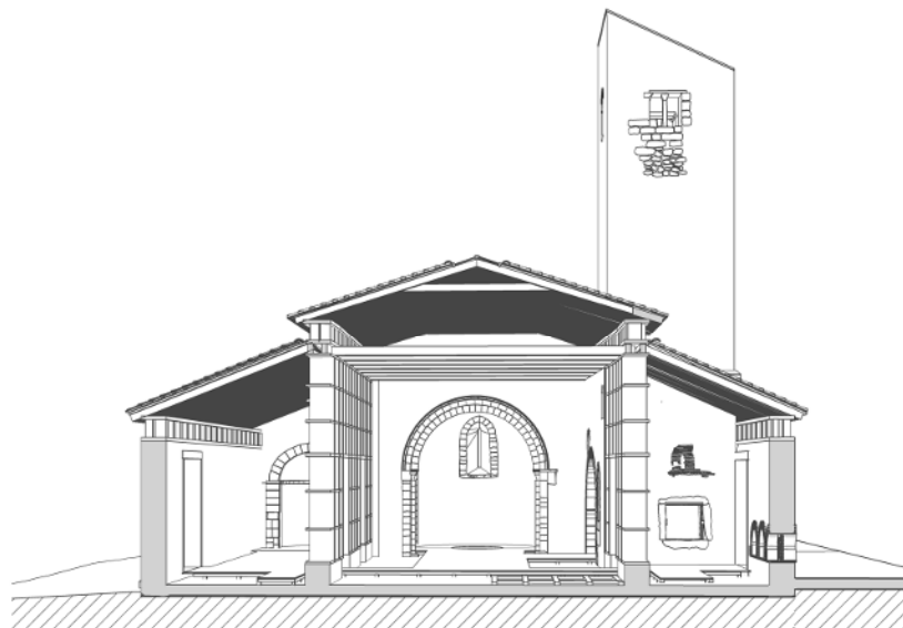
SECCION H-H
