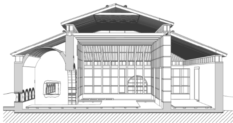
SECCION I-I
