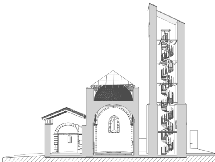
SECCION G-G
